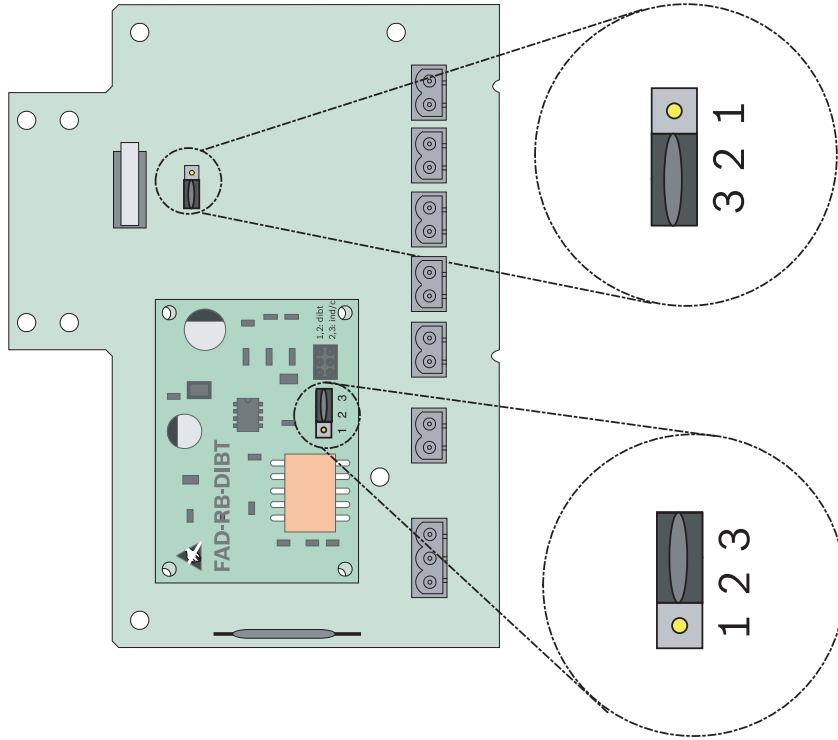
Şekil 6.1: Atlatici ayarı
