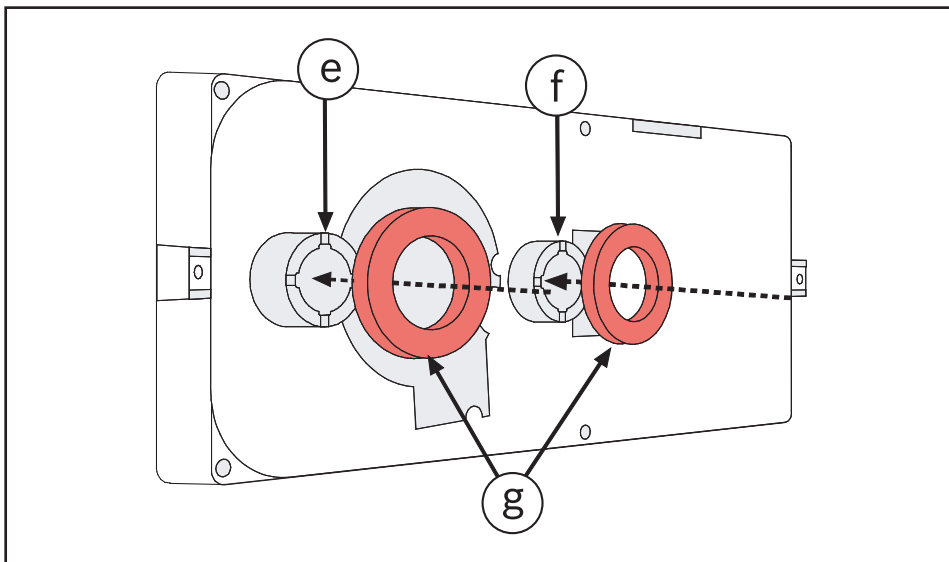
Abbildung 4.7: Dichtungsringe
