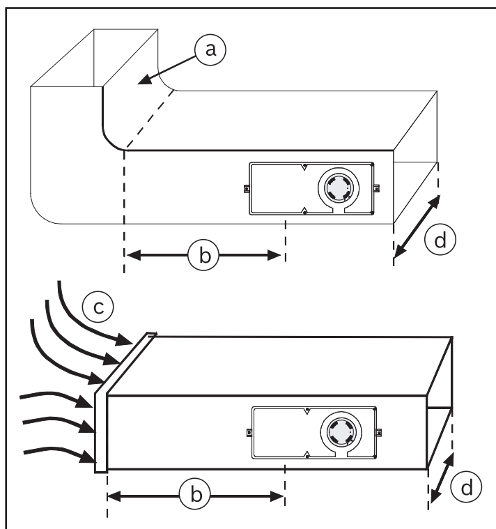
Рис. 3.1: Размещение
