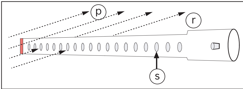
Ábra 4.10: Levegőáramlás iránya
