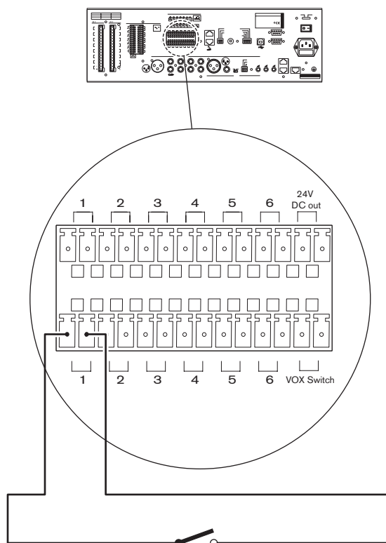
Figura 5.20: Ligar entradas de contacto para chamadas comerciais
