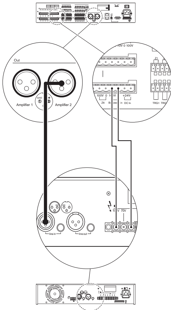
Figura 5.22: Ligar o amplificador de potência externo 2
