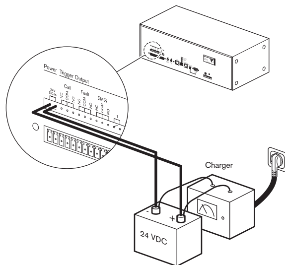
Figura 5.29: Ligar uma fonte de alimentação
