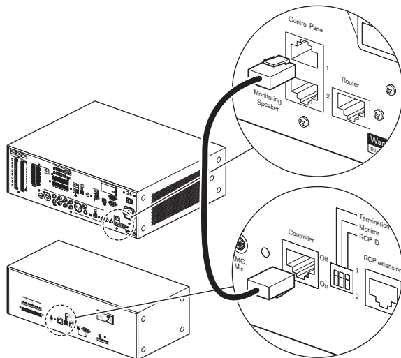
Figura 5.5: Ligar um controlo remoto
