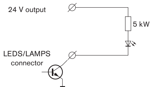
Figura 5.26: Ligar os LEDs
