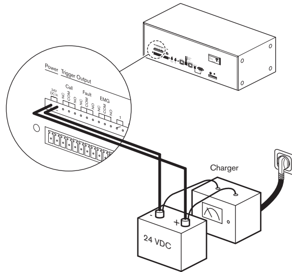
Figura 5.25: Ligar uma fonte de alimentação de 24 Vdc
