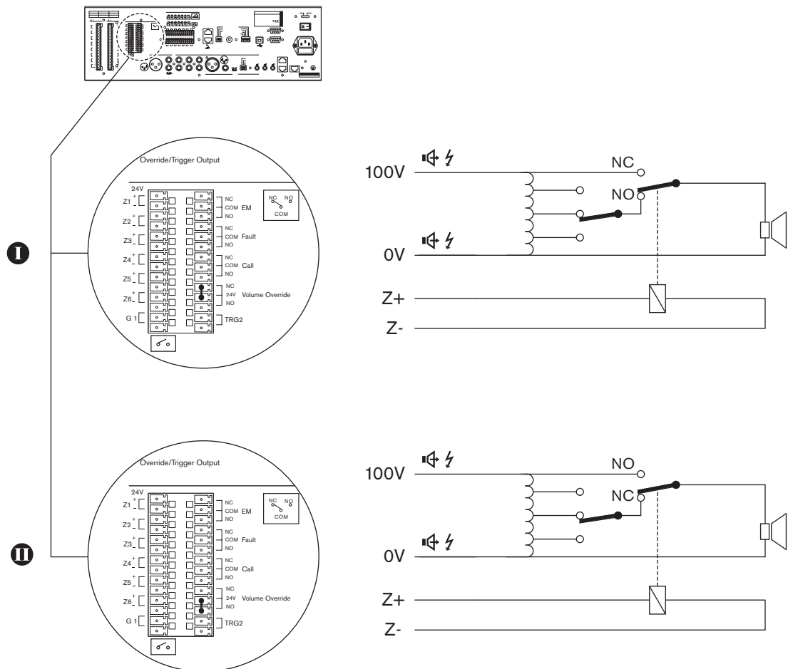
Figura 5.9: Sobreposição do regulador de volume a 4 fios
