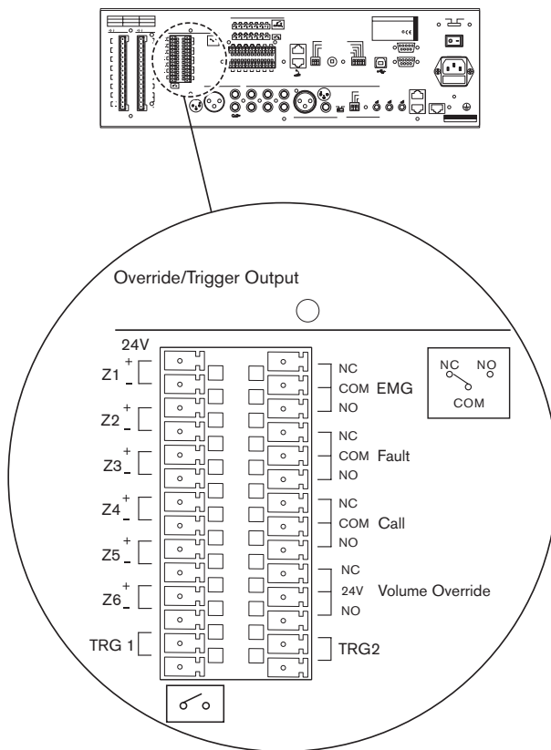
Figura 5.7: Saídas de sobreposição
