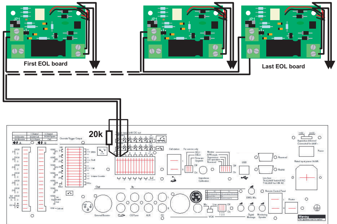
Figura 4.5: Indicação da entrada de contacto
