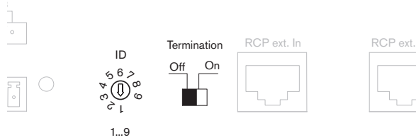
Figura 6.9: Definições do controlo remoto
