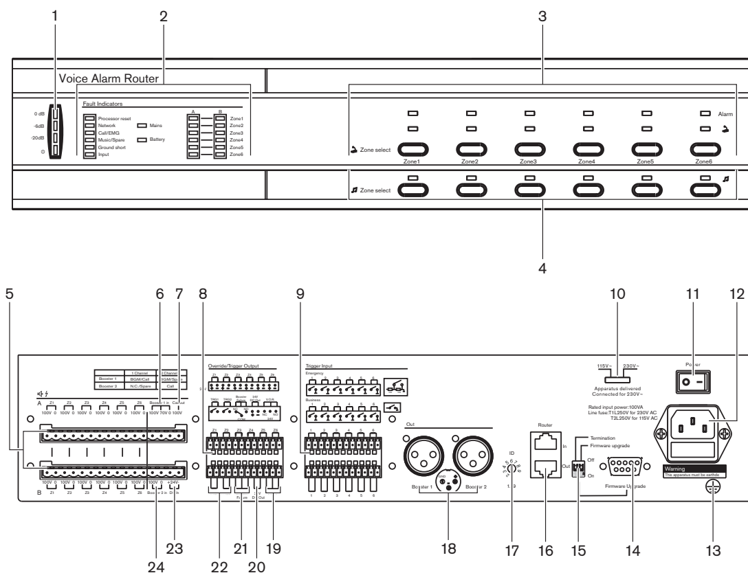
Figura 3.4: Vistas frontais e posteriores do router de alarme por voz
