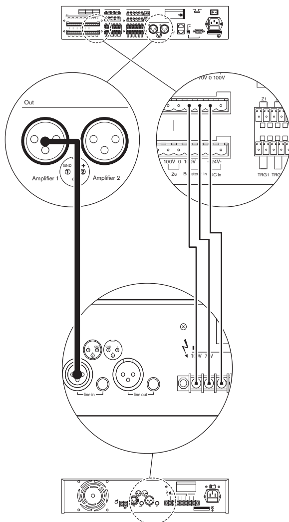
Figura 5.21: Ligar o amplificador de potência externo 1
