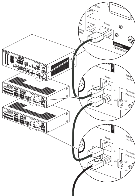
Figura 5.3: Ligar os routers
