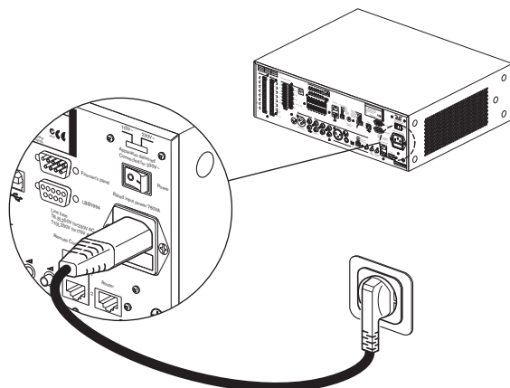
Figura 5.17: Ligar o cabo de alimentação
