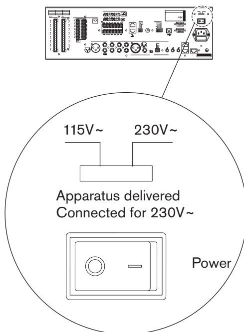
Figura 5.16: Selector de tensão
