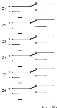
Figura 5.8: Contactos de sobreposição dos reguladores de volume
