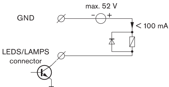
Figura 5.28: Ligar os relés
