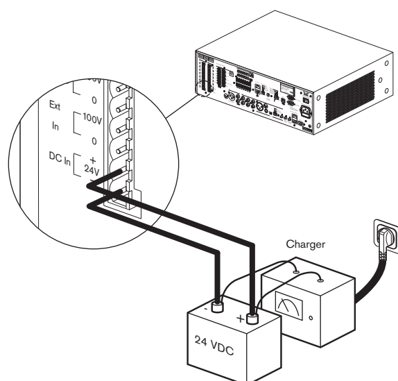
Figura 5.18: Ligar uma fonte de alimentação de reserva
