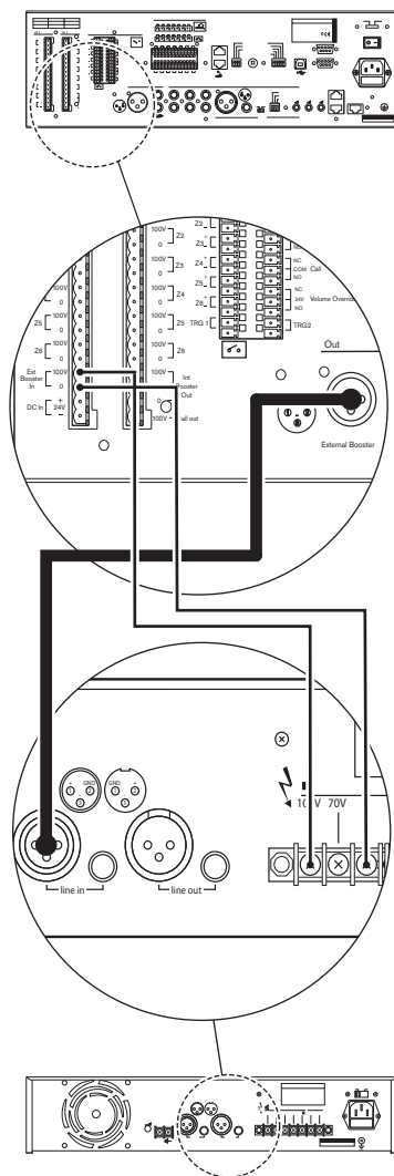
Figura 5.4: Ligar um amplificador de potência externo
