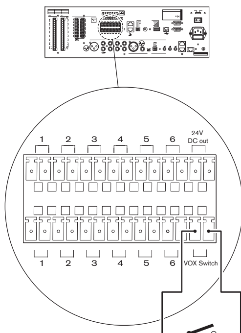
Figura 5.13: Ligar um interruptor VOX
