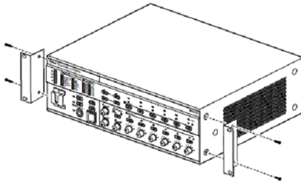
Figura 4.1: Suportes para montagem em bastidor
