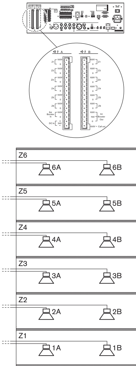
Figura 5.6: Ligar zonas de altifalantes
