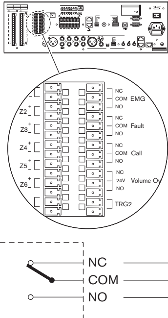
Figura 5.15: Contactos de saída de estado (por defeito)
