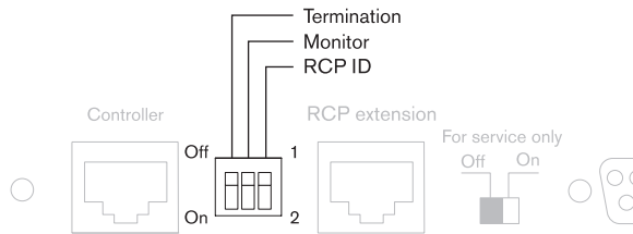
Figura 6.8: Definições do controlo remoto
