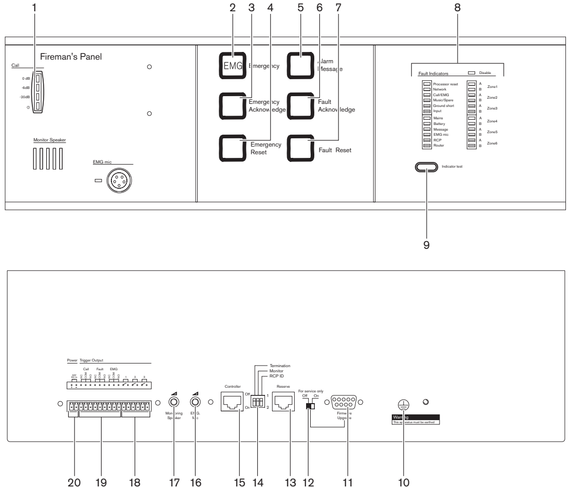
Figura 3.13: Vistas frontais e posteriores do painel para bombeiros
