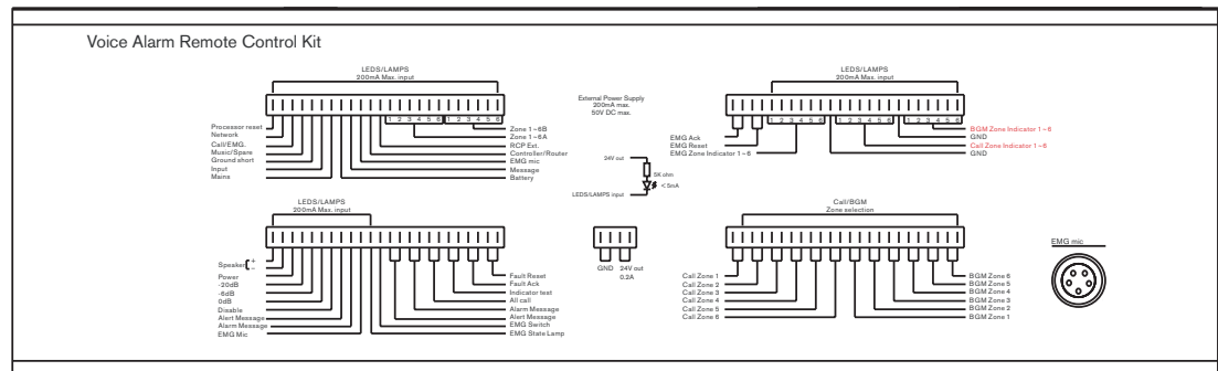
Figura 3.10: Vistas frontais e posteriores do kit de controlo remoto
