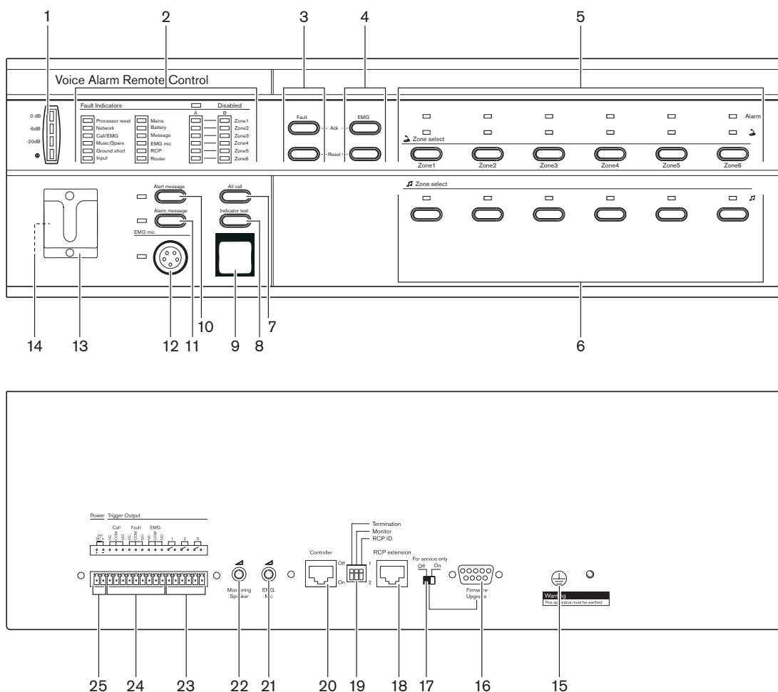
Figura 3.9: Vistas frontais e posteriores do controlo remoto de alarme por voz
