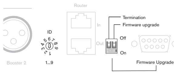
Figura 6.6: Definições do Router
