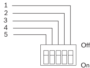
Figura 6.1: Interruptores DIP para definições do sistema
