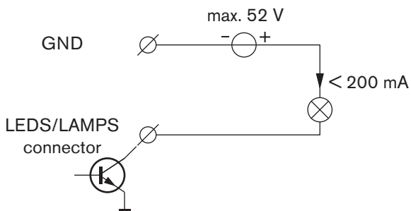
Figura 5.27: Ligar as lâmpadas
