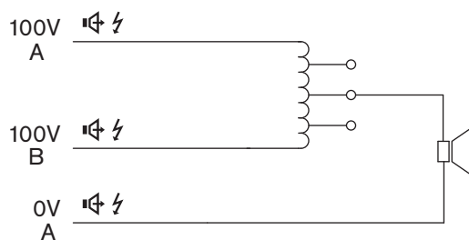
Figura 5.10: Sobreposição do regulador de volume a 3 fios
